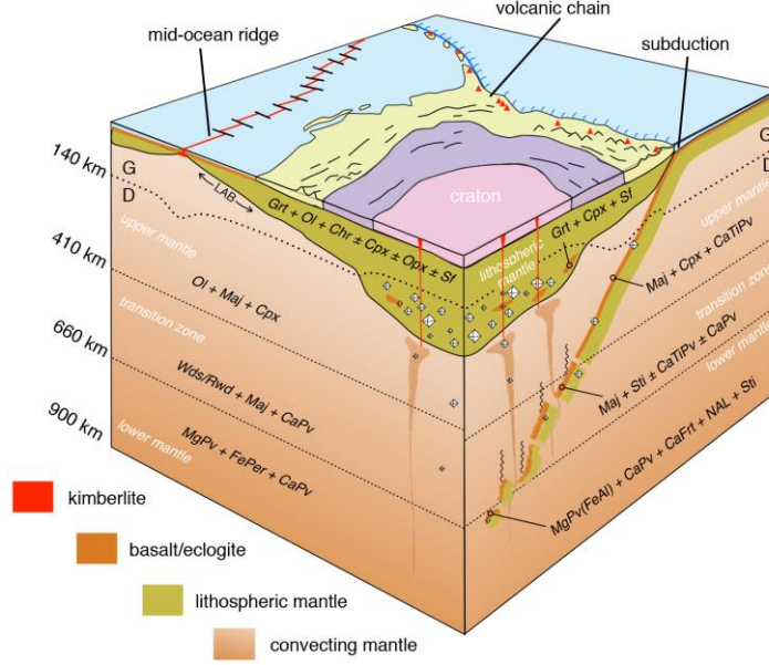
Resim 2. Konveksiyonel Manto, Dünyanın İç Elmas Oluşum Bölgeleri. G:Grafite, D: Elmas, (Shirey, S, vd., 2013:358)
