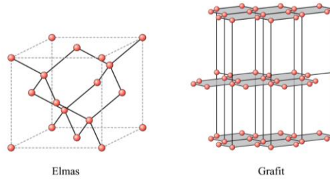
Resim 1. Elmas ve Grafitin Kristal Yapısı (R. Tappert, M.C. Tappert, 2011:1)
