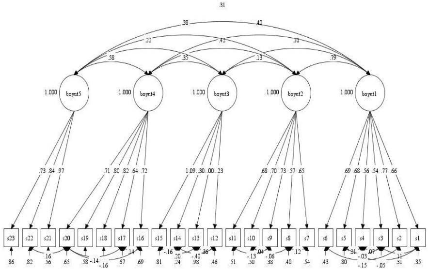
Şekil 1. Bilgi ve İletişim Teknolojileri (BİT) Tutum Ölçeğinin Doğrulayıcı Faktör Analizi Sonucu Elde Edilen Path Diyagramı
